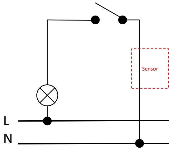
Schaltkreis 1
