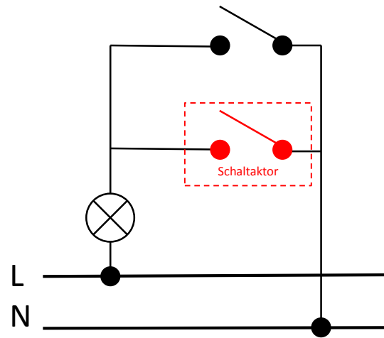
Schaltkreis 2
