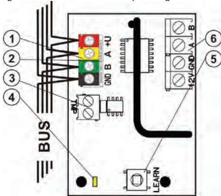
Abbildung 1: 1 – Bus-Klemmen; 2 – Seriennummer auf der Seite der Klemmleiste; 3 – TMP-Klemme; 4 – gelbe LED; 5 – LEARN-Taste (Tamper – Feder ist im Lieferumfang enthalten); 6 – RS-485-Schnittstelle
