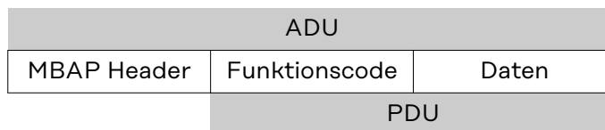
Struktur einer Modbus Nachricht bei Modbus TCP
